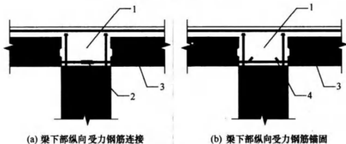
图 7.3.8-3 预制柱及叠合梁框架顶层中节点构造示意 1—后浇区；2—梁下部纵向受力钢筋连接； 3—预制梁；4—梁下部纵向受力钢筋锚固
