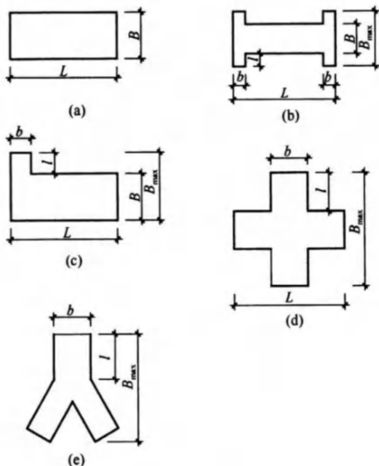
图 6.1.5 建筑平面示例
