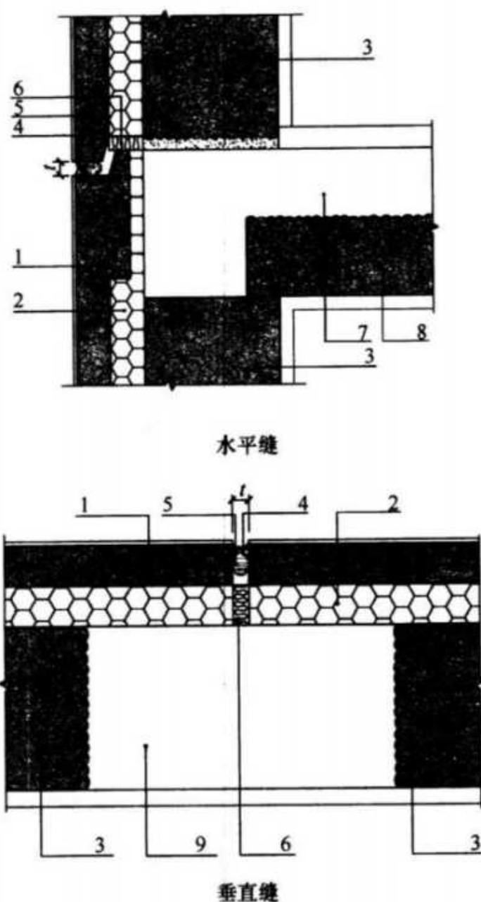
图1 预制承重夹心外墙板接缝构造示意
