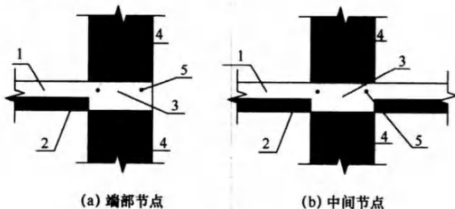
图 8.3.3 水平后浇带构造示意
