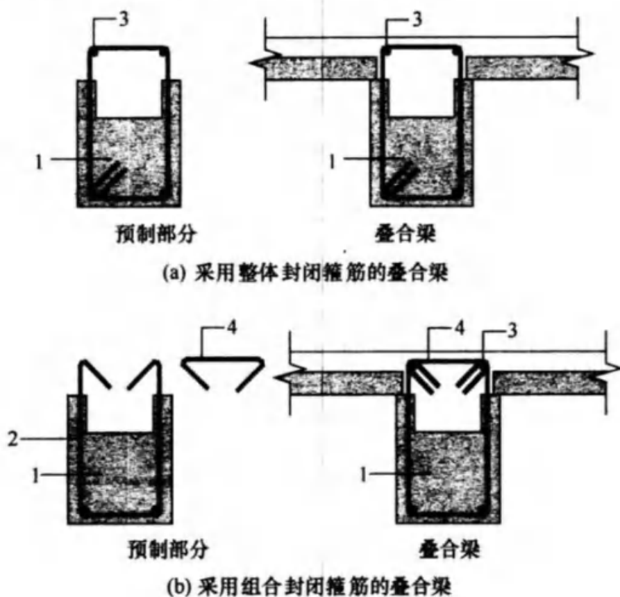
图 7.3.2 叠合梁箍筋构造示意
