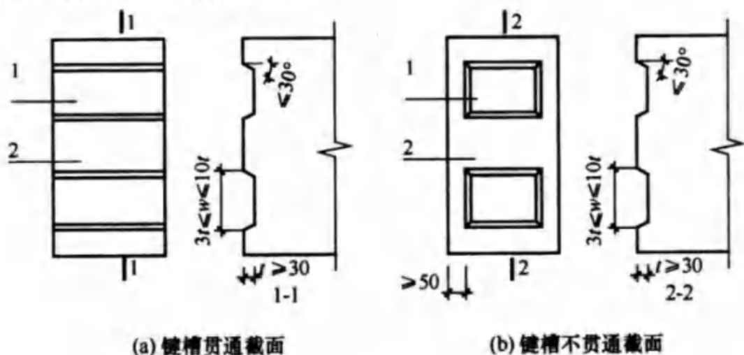
图 6.5.5 梁端键槽构造示意 1—键槽；2—梁端面
