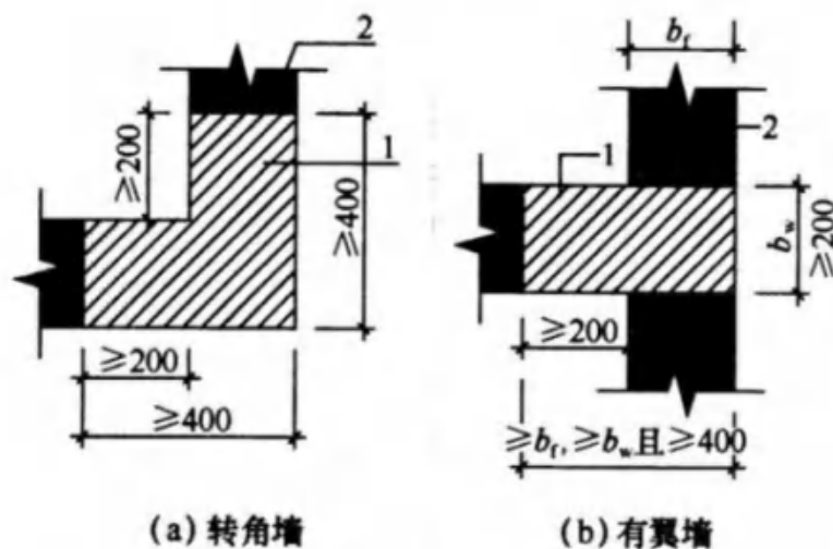
图 8.3.1-2 构造边缘构件全部后浇构造示意 (阴影区域为构造边缘构件范围)
