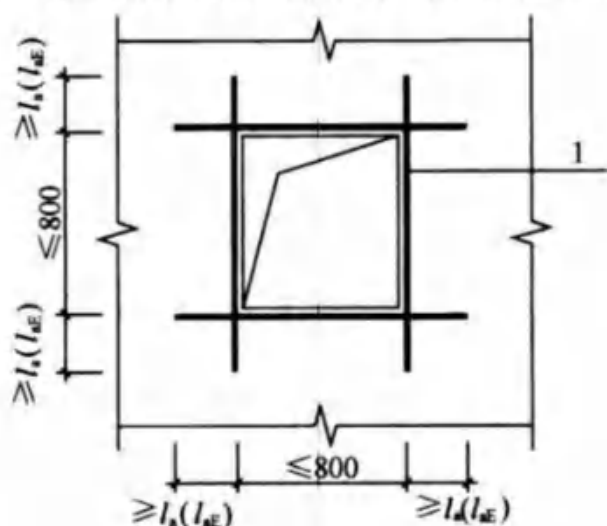
图 8.2.3 预制剪力墙洞口补强钢筋配置示意
