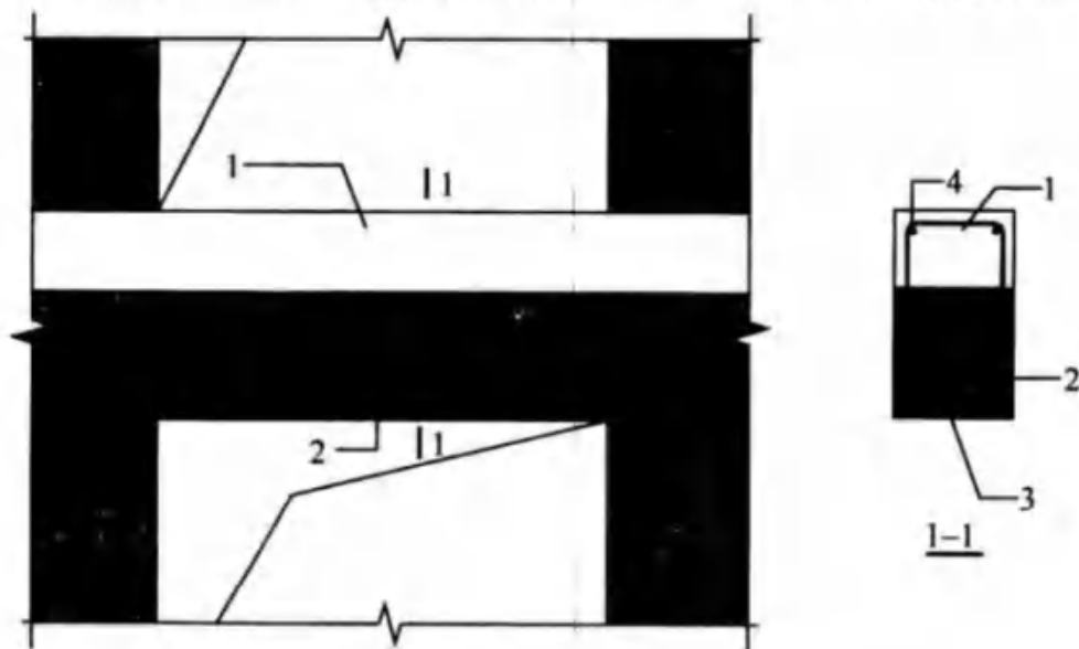
图 8.3.8 预制剪力墙叠合连梁构造示意
