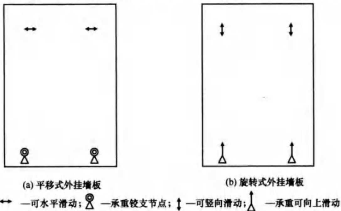
图 6 外挂墙板及其连接节点形式示意
