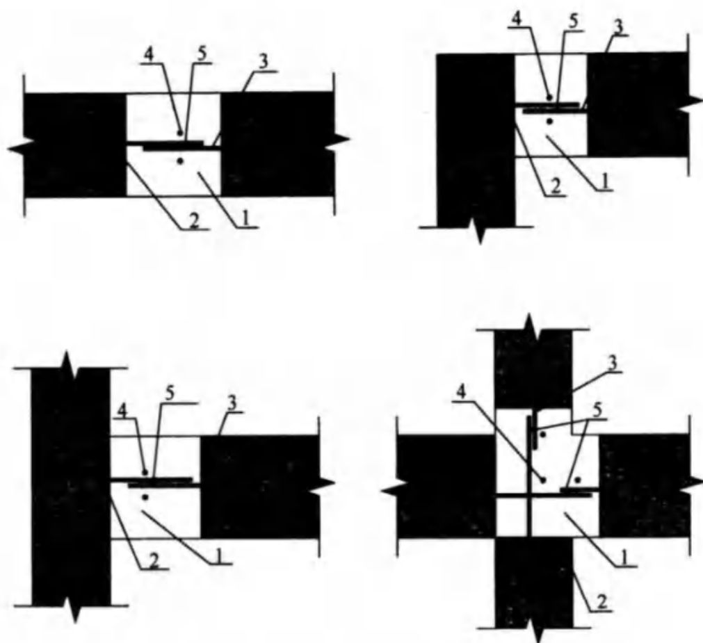
图5 预制墙板竖向接缝构造示意
