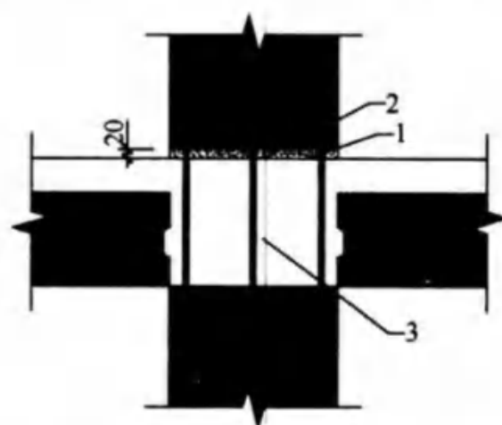
图 7.3.6 预制柱底接缝构造示意
