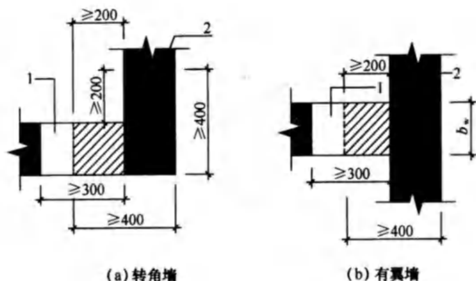
图 8.3.1-3 构造边缘构件部分后浇构造示意 (阴影区域为构造边缘构件范围)
