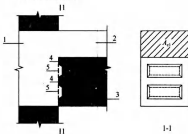
图 7.2.2 叠合梁端受剪承载力计算参数示意
