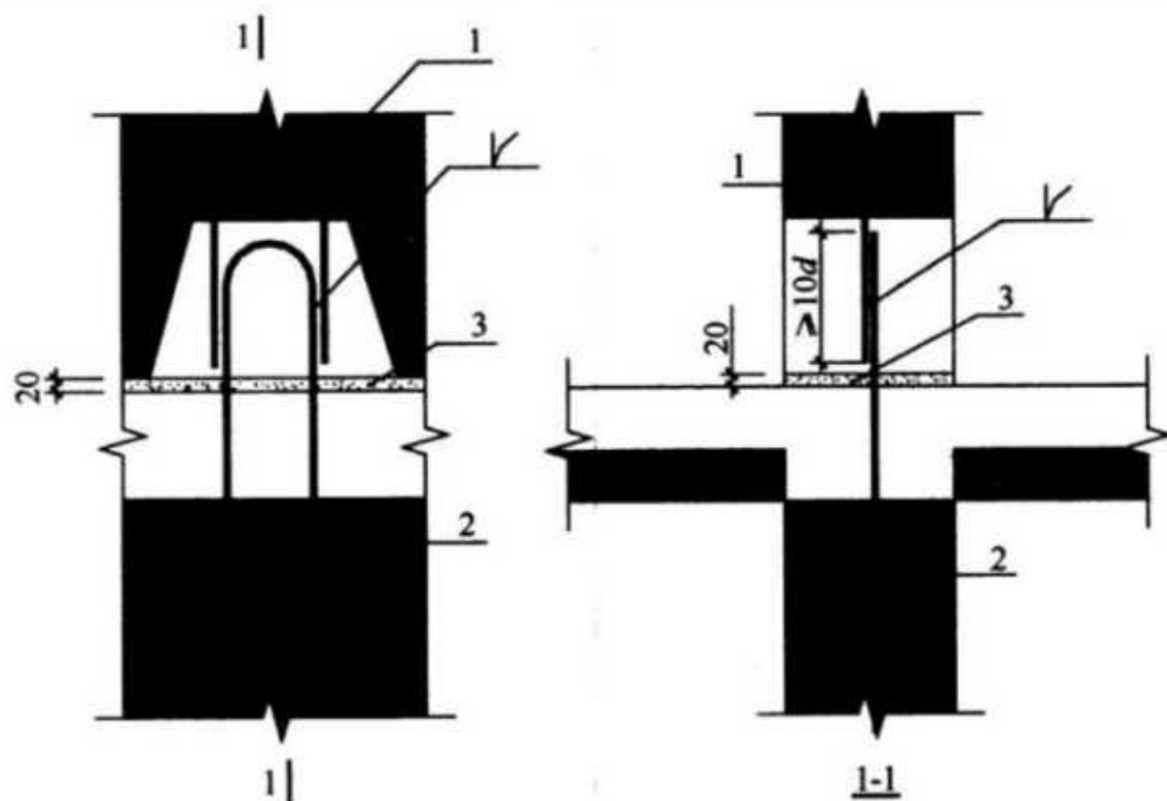
图 A.0.3 连接钢筋焊接连接构造示意
