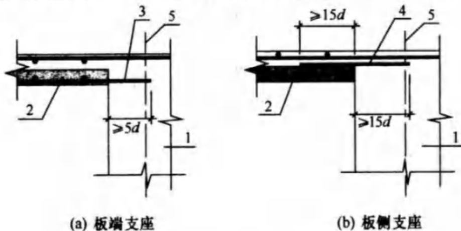
图 6.6.4 叠合板端及板侧支座构造示意
