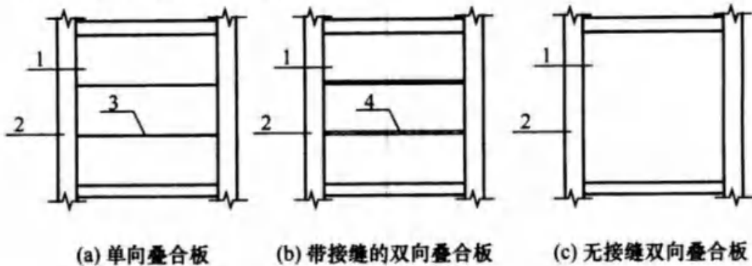
图 6.6.3 叠合板的预制板布置形式示意
