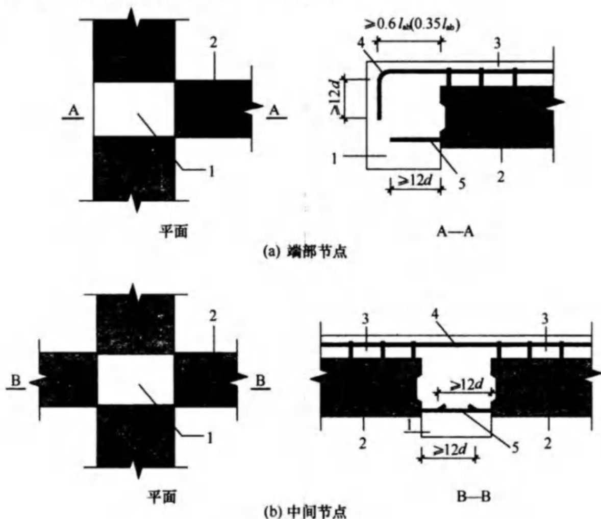
图 7.3.4 主次梁连接节点构造示意
