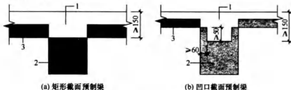
图 7.3.1 叠合框架梁截面示意
