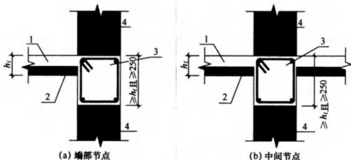
图 8.3.2 后浇钢筋混凝土圈梁构造示意
