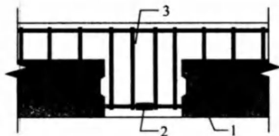
图 7.3.3 叠合梁连接节点示意
